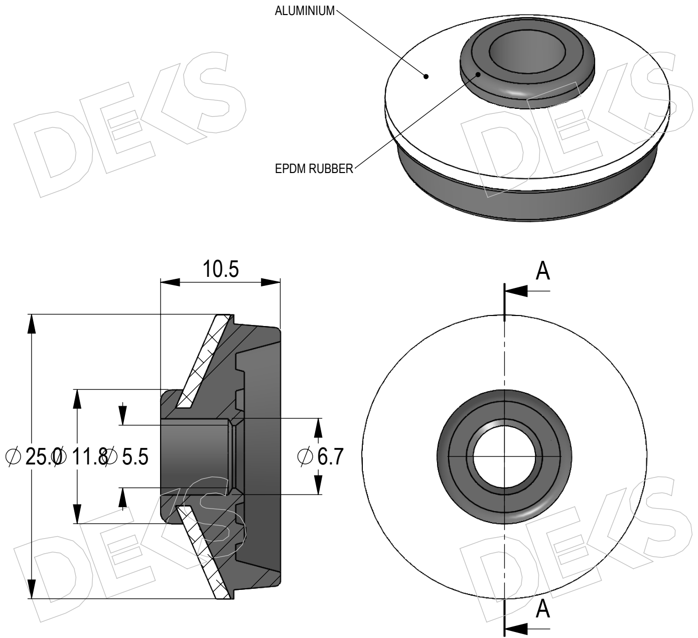
SECTION A-A
