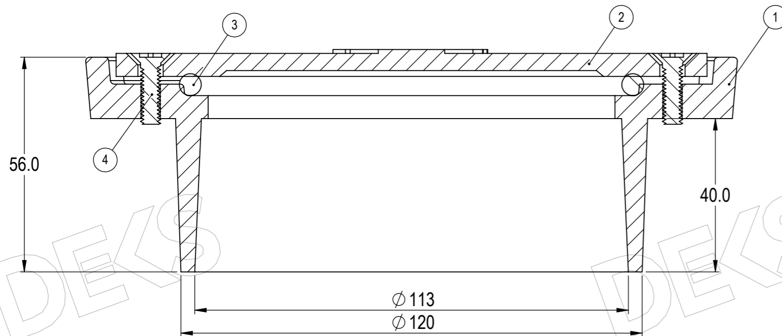
SECTION A-A
